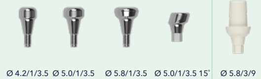
Ø 4.2/1/3.5 Ø 5.0/1/3.5 Ø 5.8/1/3.5 Ø 5.0/1/3.5 15° Ø 5.8/3/9
